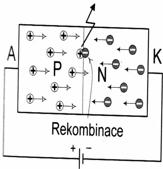
~ PN přechod homogenní
