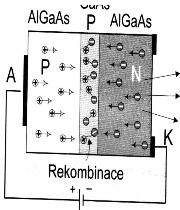
PN přechod heterogenní
