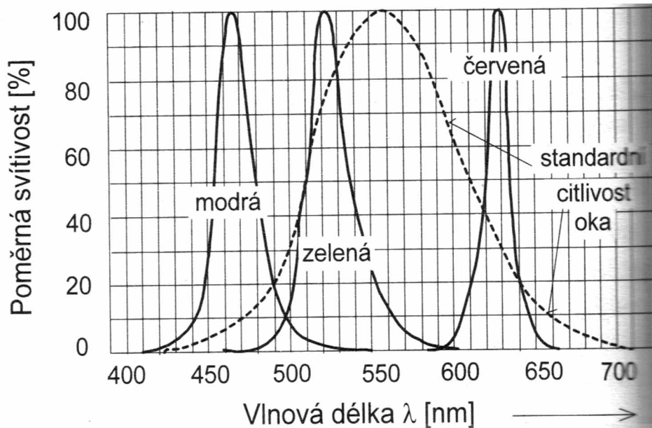
spektrální garakteristiky LED
